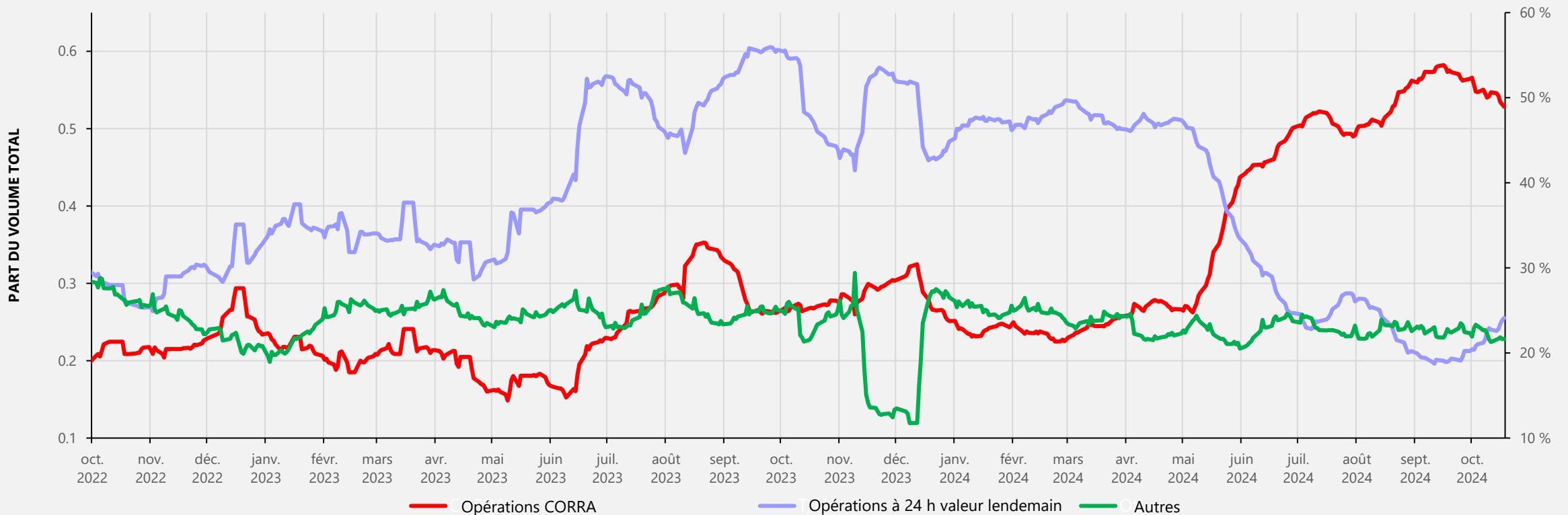
Graphique 9 : Moyenne mobile sur 20 jours de la part des opérations de pension selon l'admissibilité pour le taux CORRA
