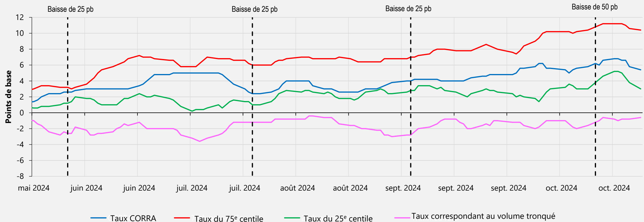
Graphique 3 : Écart par rapport au taux cible de la moyenne mobile sur 5 jours du taux CORRA, des centiles et du taux correspondant au volume tronqué
