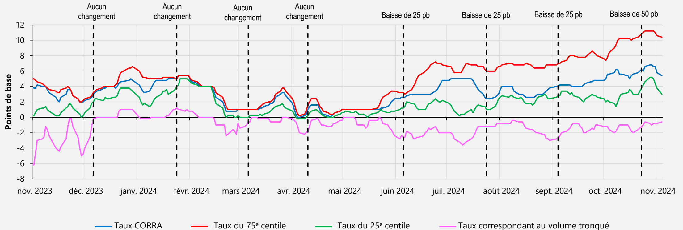
Graphique 1 : Écart par rapport au taux cible de la moyenne mobile sur 5 jours du taux CORRA, des centiles et du taux correspondant au volume tronqué
