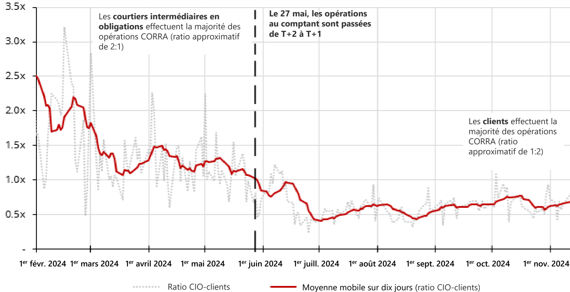
Graphique 10 : Ratio entre les opérations effectuées par des courtiers intermédiaires en obligations (CIO) et celles par des clients (volume des opérations de pension à un jour, montant réglé)
