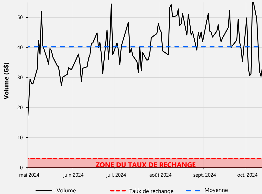
Graphique 7 : Volume quotidien d'opérations CORRA depuis le 28 mai 2024
