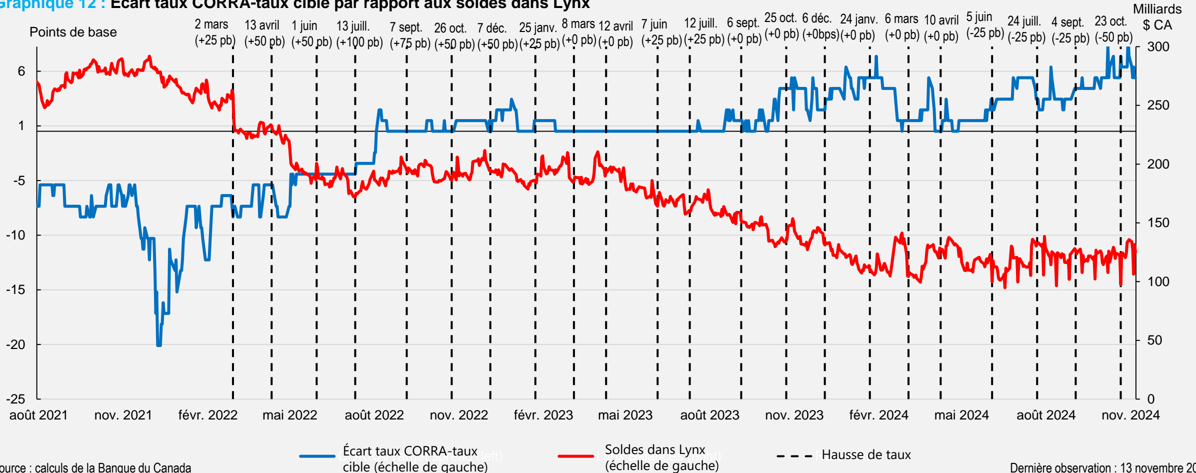
Graphique 12 : Écart taux CORRA-taux cible par rapport aux soldes dans Lynx
