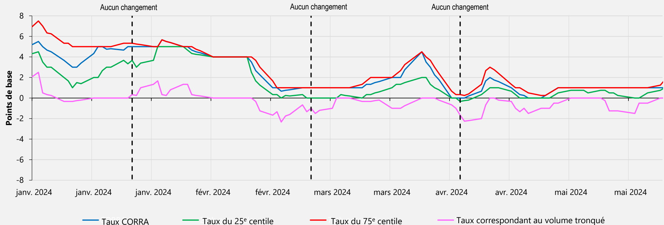
Graphique 2 : Écart par rapport au taux cible de la moyenne mobile sur 5 jours du taux CORRA, des centiles et du taux correspondant au volume tronqué
