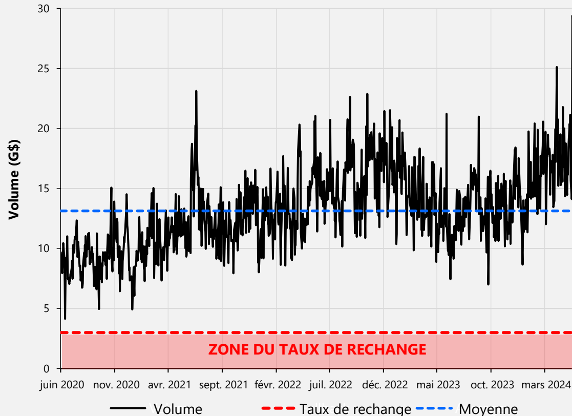
Graphique 5 : Volume quotidien d'opérations CORRA depuis juin 2020
